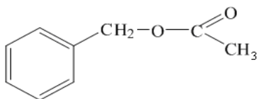
бензилацетат
