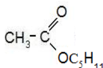
изоамилацетат
