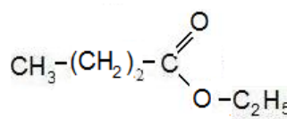
этилбутират
